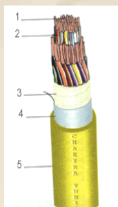
TELECOM CABLE 5/9 NFC 93-527-12
